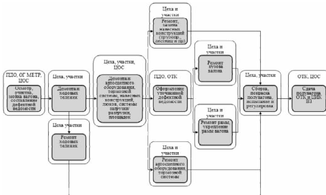
Рис. 1. Схема технологического процесса ремонта полувагона
