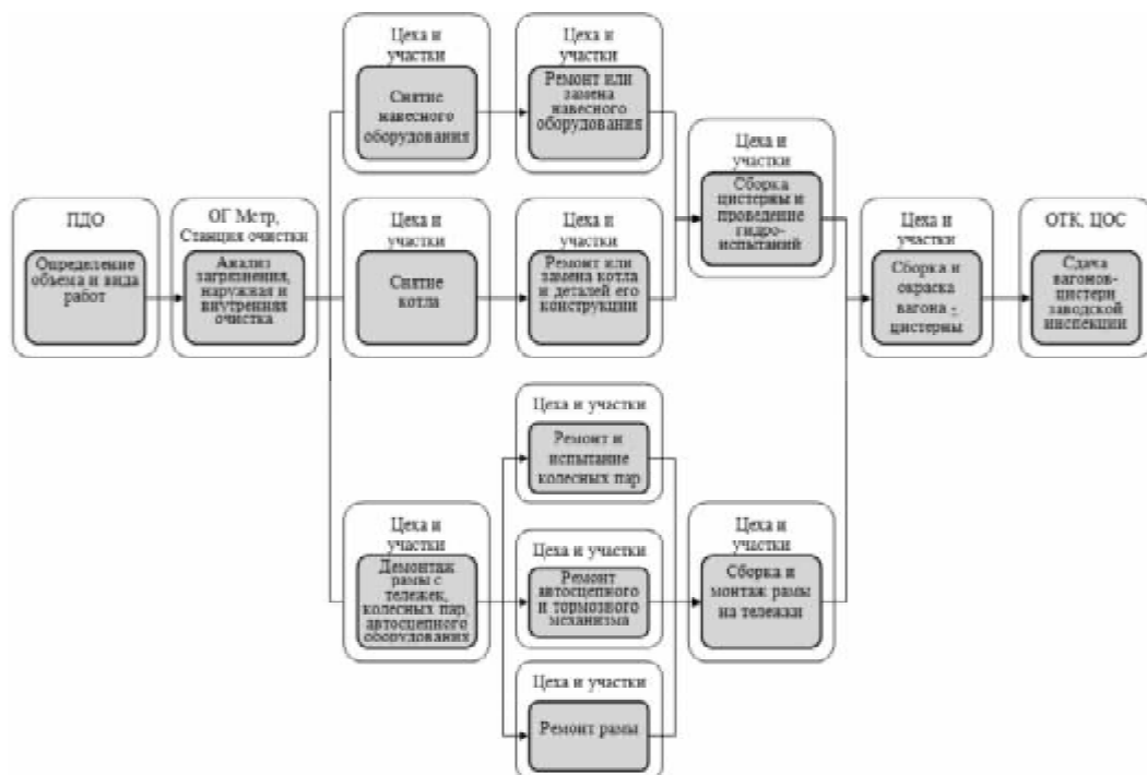
Рис. 2. Схема технологического процесса ремонта вагона-цистерны
